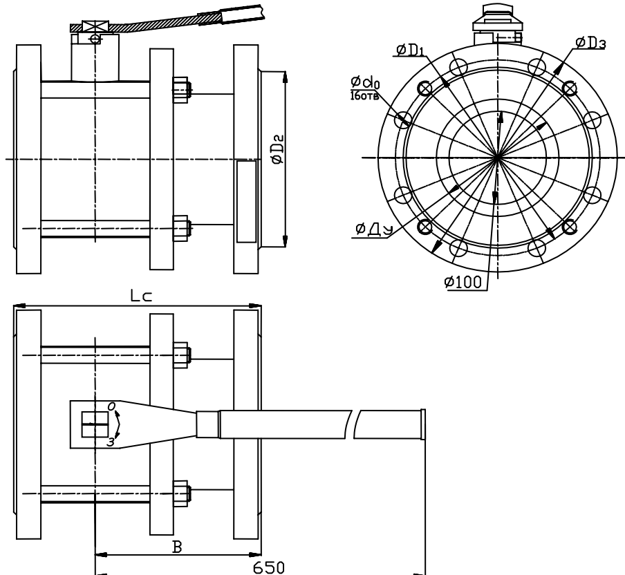
Рисунок 1. Общий вид крана
