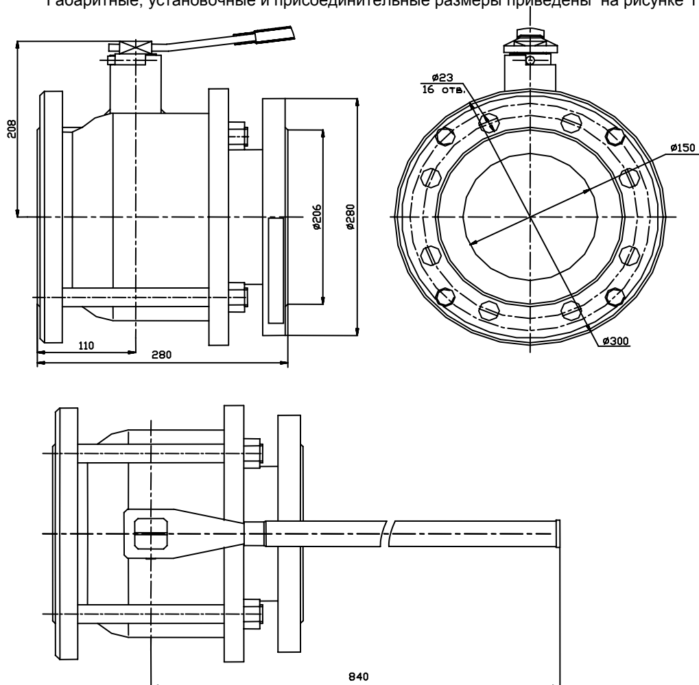
Рисунок 1. Общий вид крана
